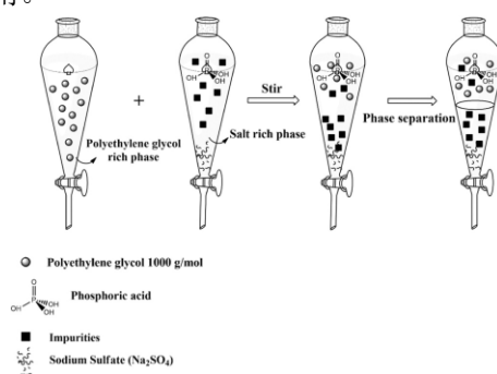
图 2 磷酸 ATPS 萃取示意图 [62]
