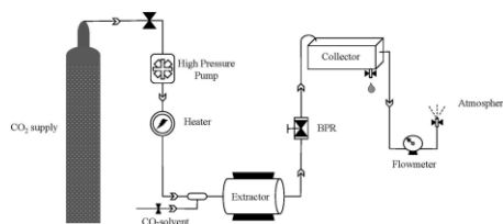
图5 超临界流体萃取之流程图 [76]
