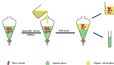
图 1 溶剂萃取原理 [8]
