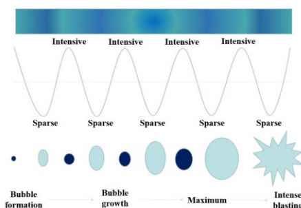
图4 超声空化过程示意图 [72]
